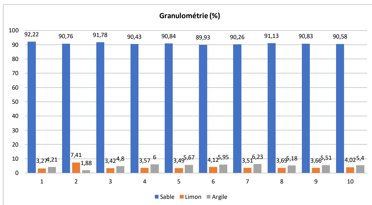
Figure 9. Granulométrie (%).
